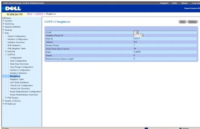
Abbildung 11-25. OSPFv3-Nachbarschaften
