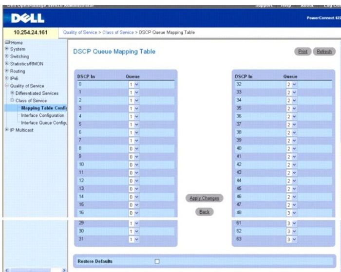
Abbildung 12-17. DSCP-Warteschlangen-Zuweisungstabelle
