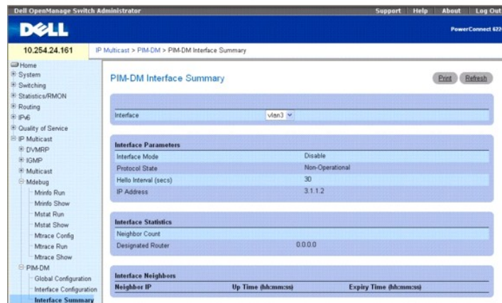
Abbildung 13-25. PIM-DM-Schnittstellen-Übersicht
